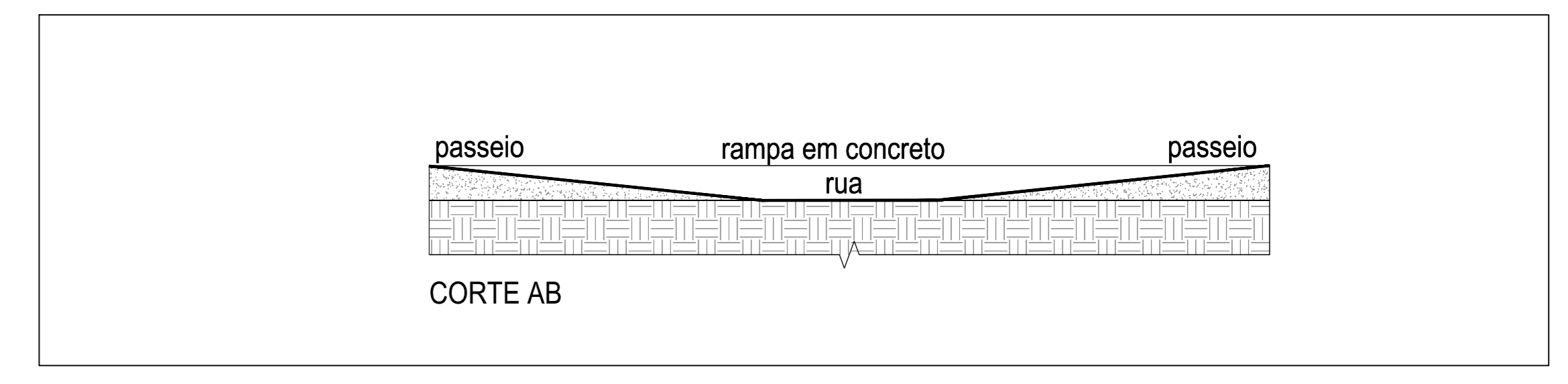
DETALHE - RAMPA DE ACESSIBILIDADE PNE - S/ ESCALA
